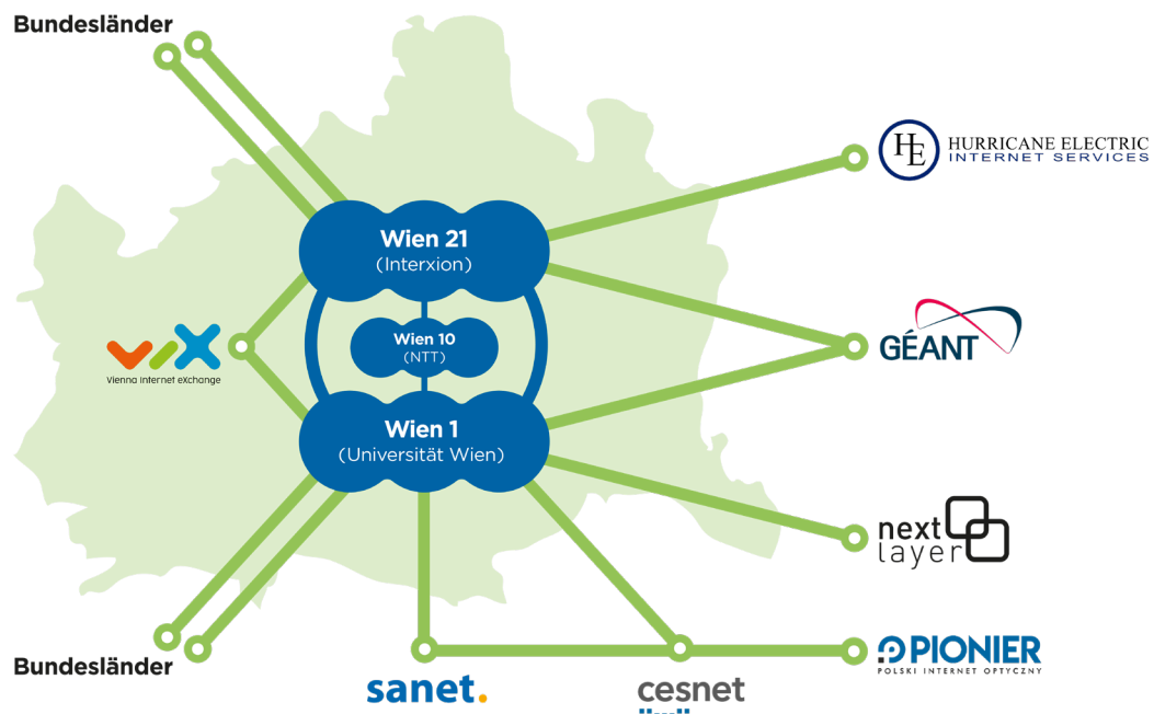
Nationale und internationale Anbindungen an den Core-Standorten von ACOnet in Wien (Stand Oktober 2022, Grafik: ACOnet / Goran Golik)
